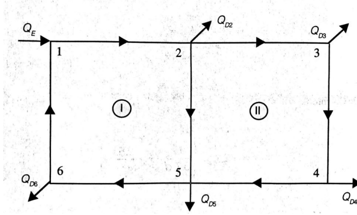
Figure 14: Red cerrada que ilustra el uso del método de programación lineal (tomado de [1]).
